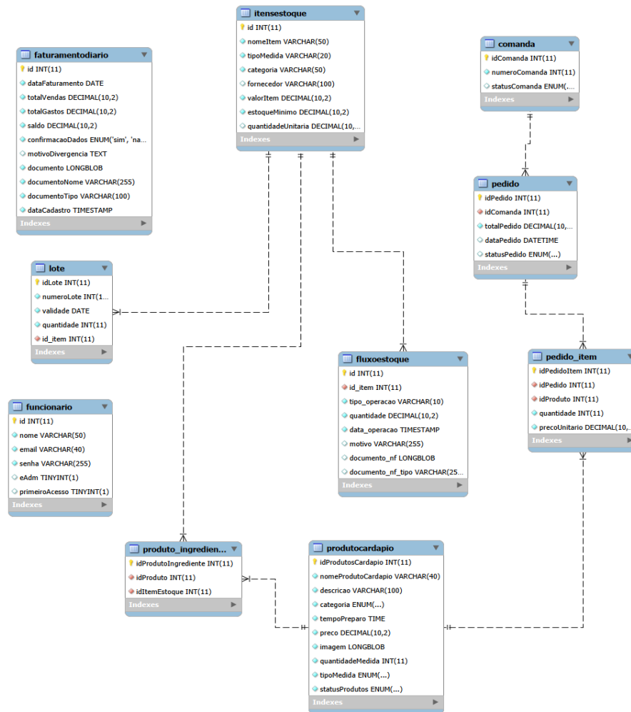
Figura 24 – Exemplo: Modelo Relacional gerado por engenharia reversa (MySQL Workbench).
